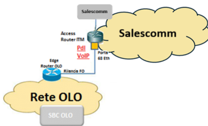
Figura 1: Modello dei punti di interconnessione VoIP
